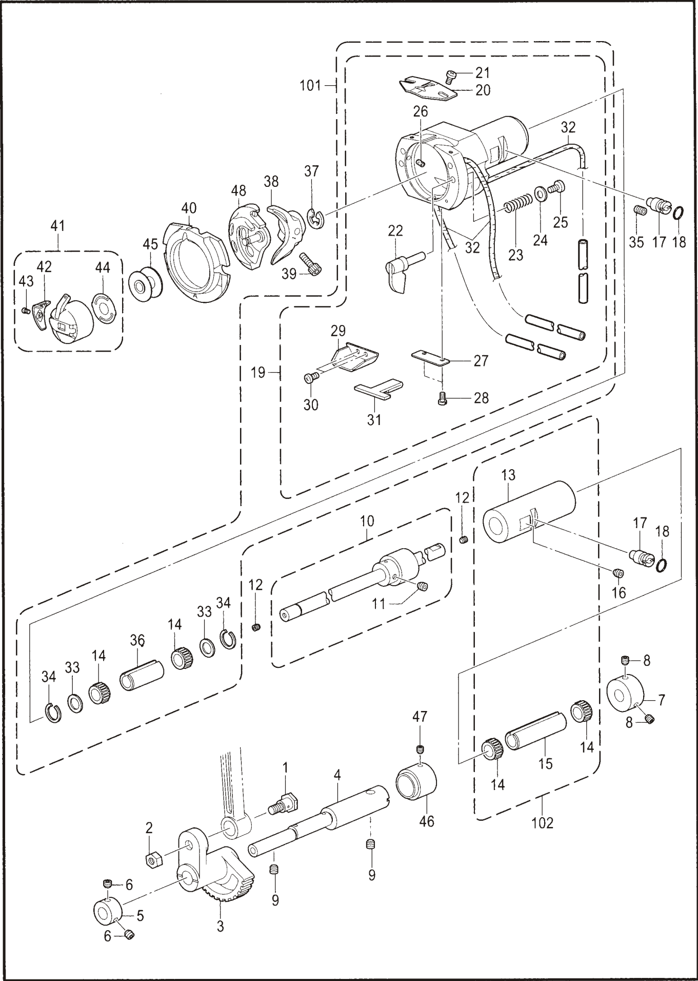
F. 下轴装置 / Lower shaft mechanism
