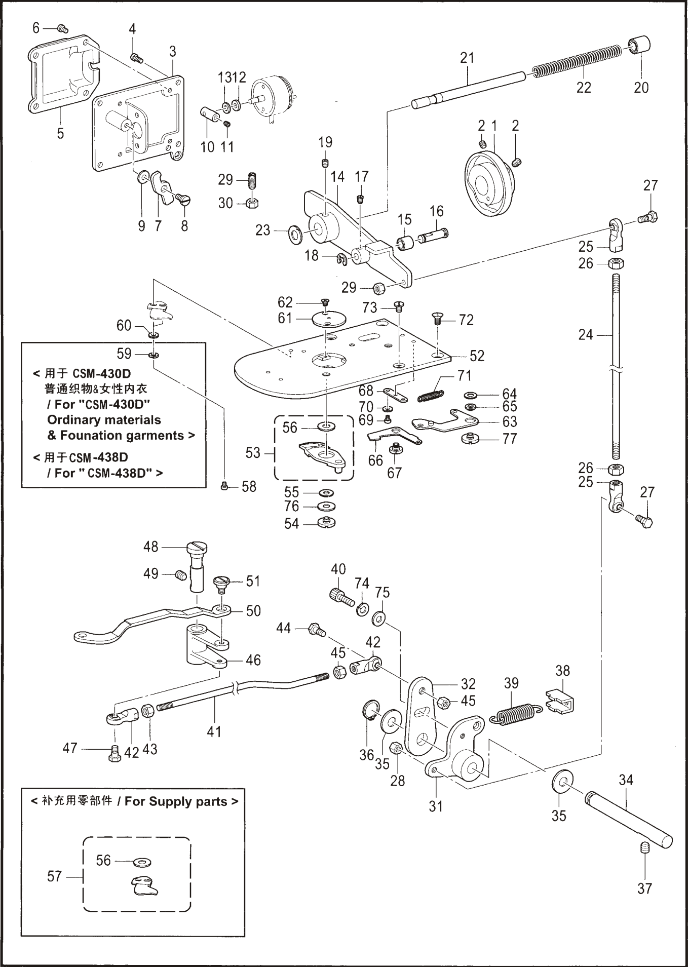
K. 切线装置 / Thread trimmer mechanism
