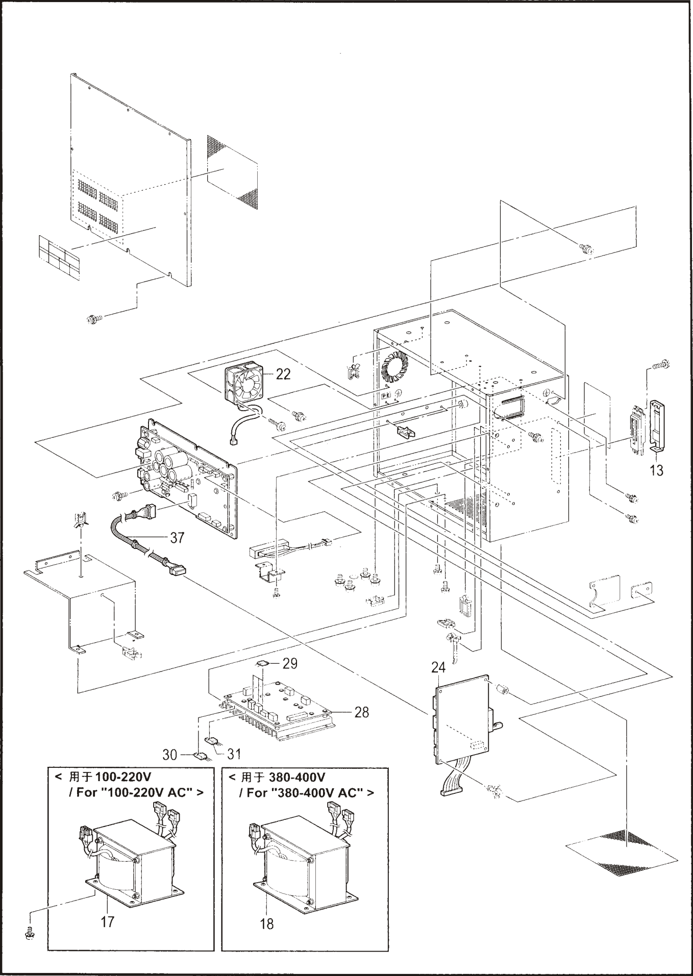
P1. 控制箱装置 / Control box mechanism
