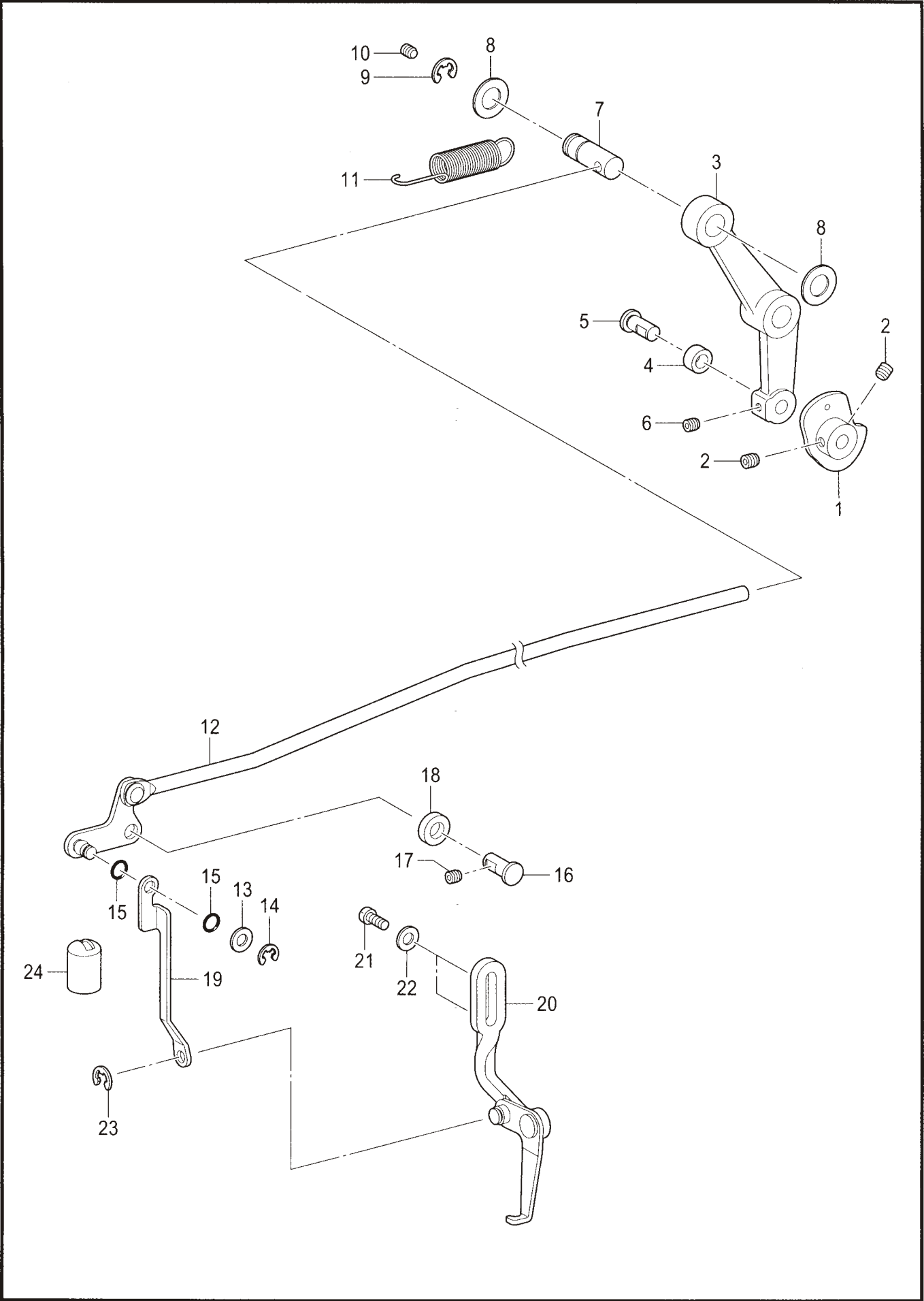
L. 扫线装置 / Thread wiper mechanism
