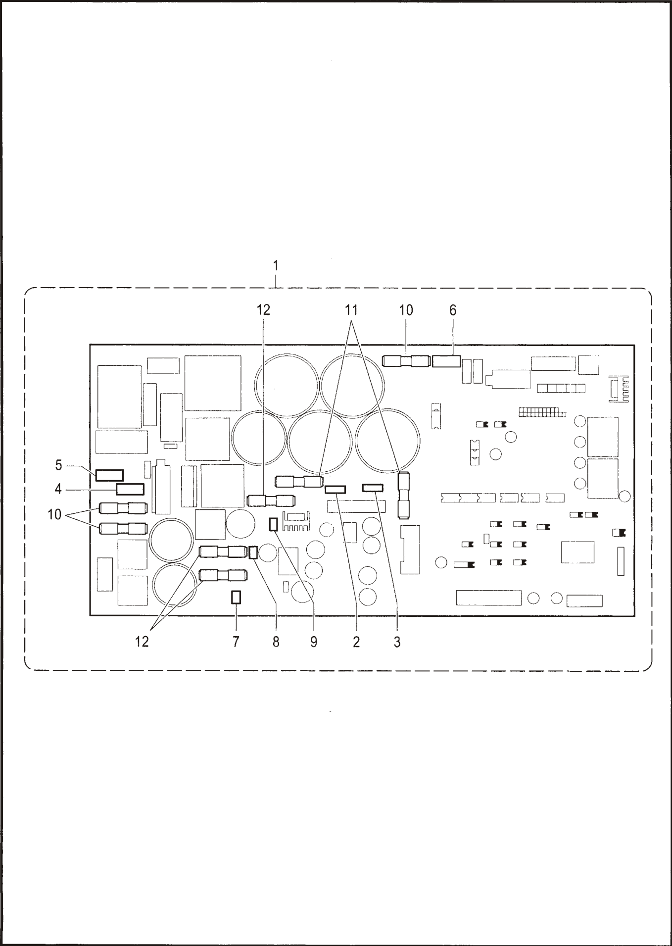
P2 . 控制箱装置(电源基板) / Control box (PCB) mechanism
